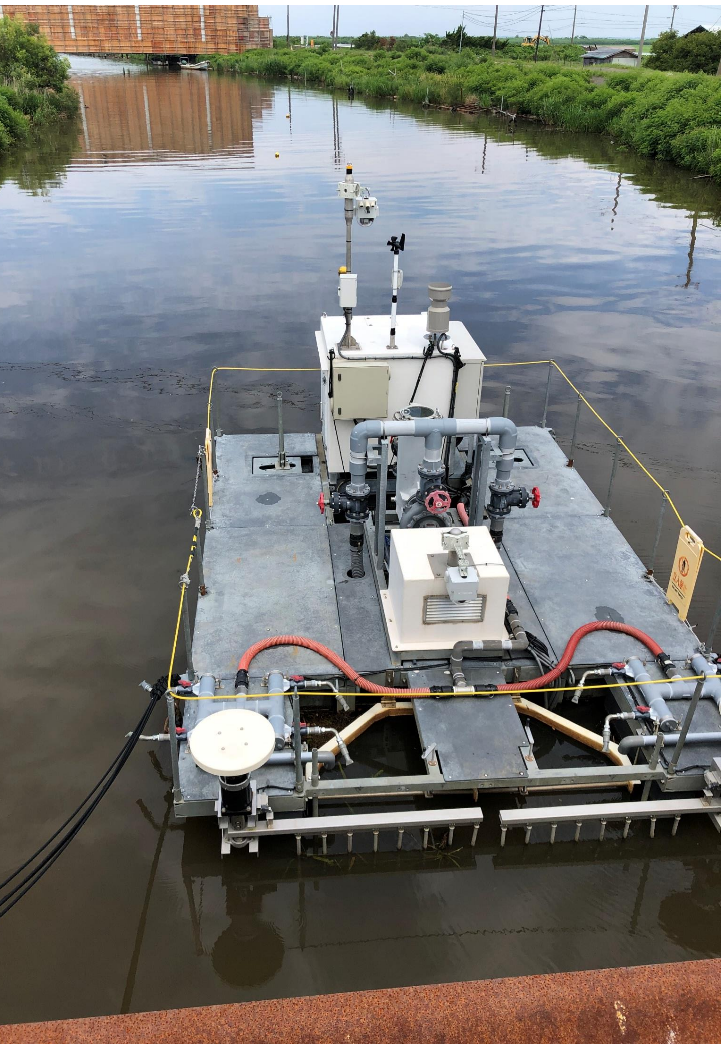
2019年度秋田県馬踏川 アオコ抑制装置
